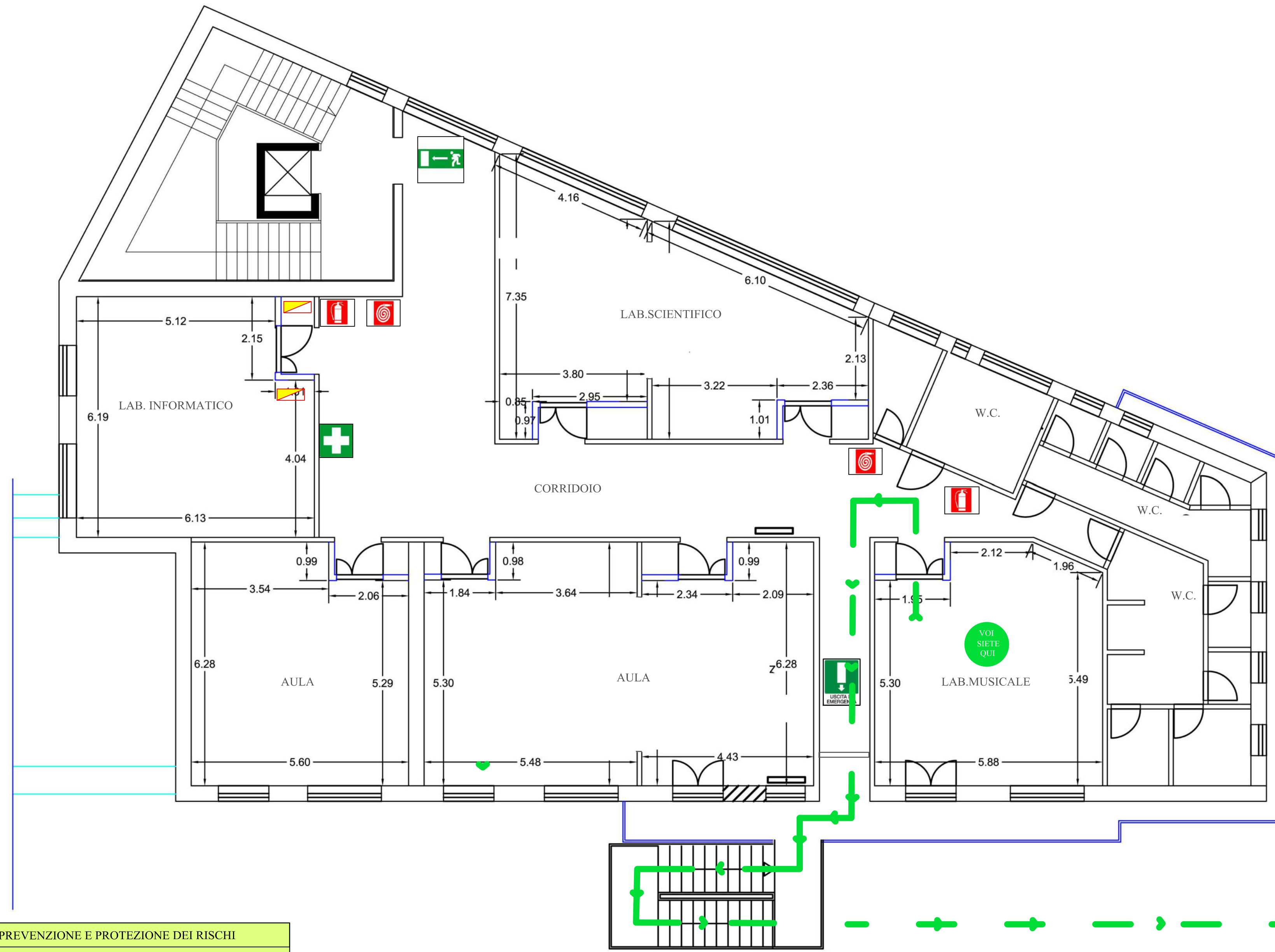
PIANTA PIANO TERZO
